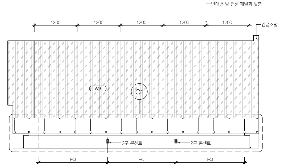
04 라운지 B104 SCALE 1:50
