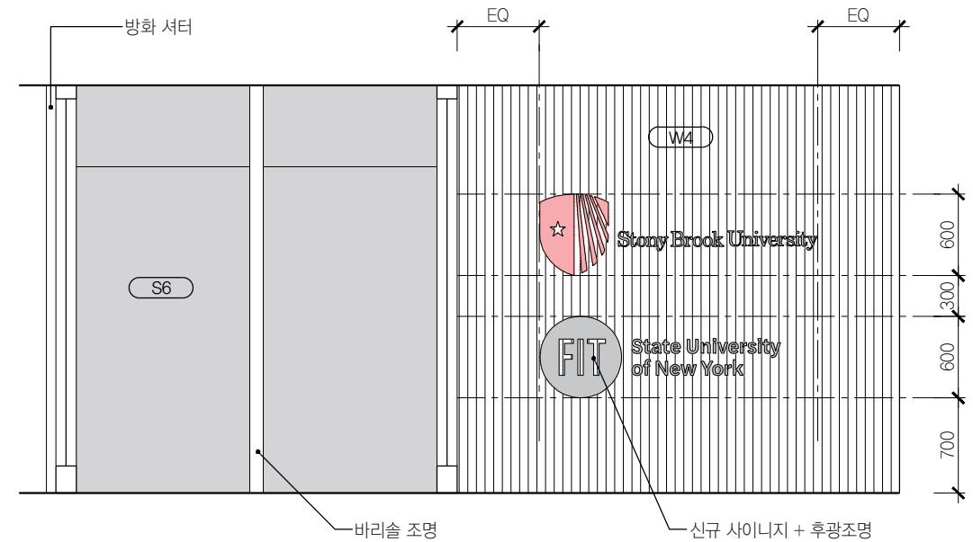
04 방풍실2 B105 SCALE 1:50
