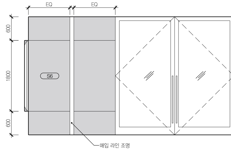
01 방풍실 B101 SCALE 1:50
