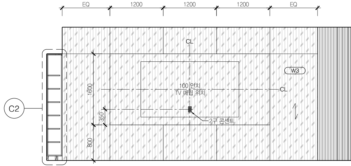
02 라운지 B104 SCALE 1:50
