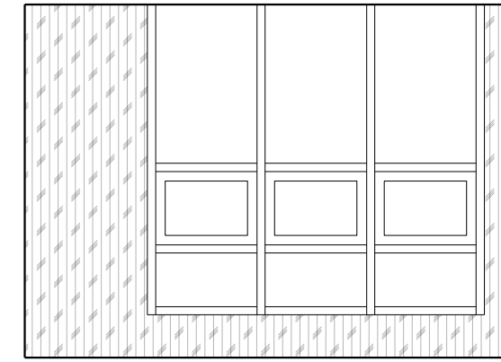
02 엘리베이터 B114 SCALE 1:50
