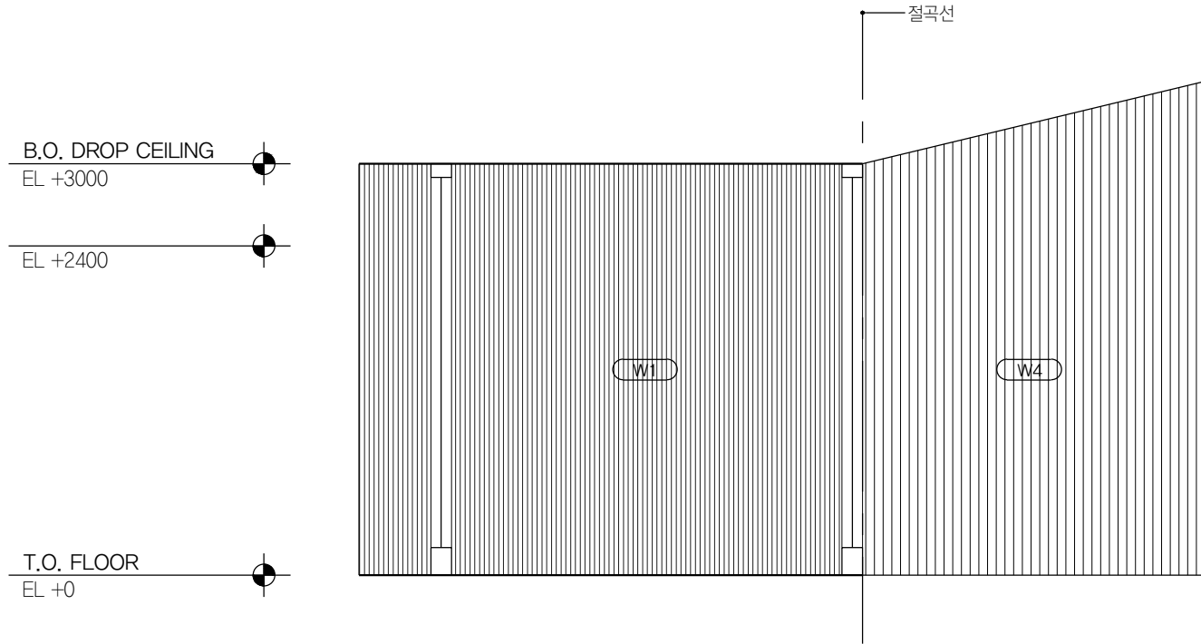
01 방풍실 B101 SCALE 1:50
