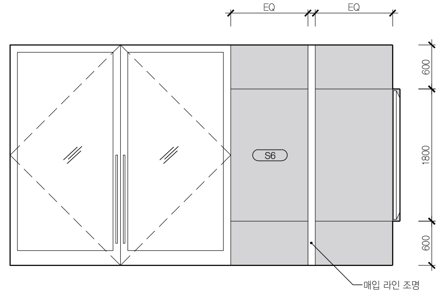
01 방풍실 B101 SCALE 1:50
