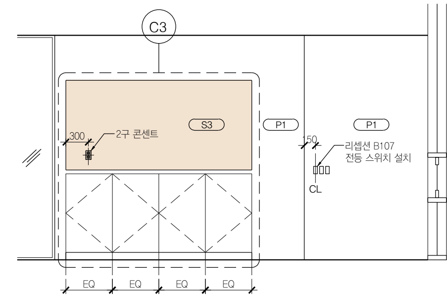
04 리셉션 B107 SCALE 1:50
