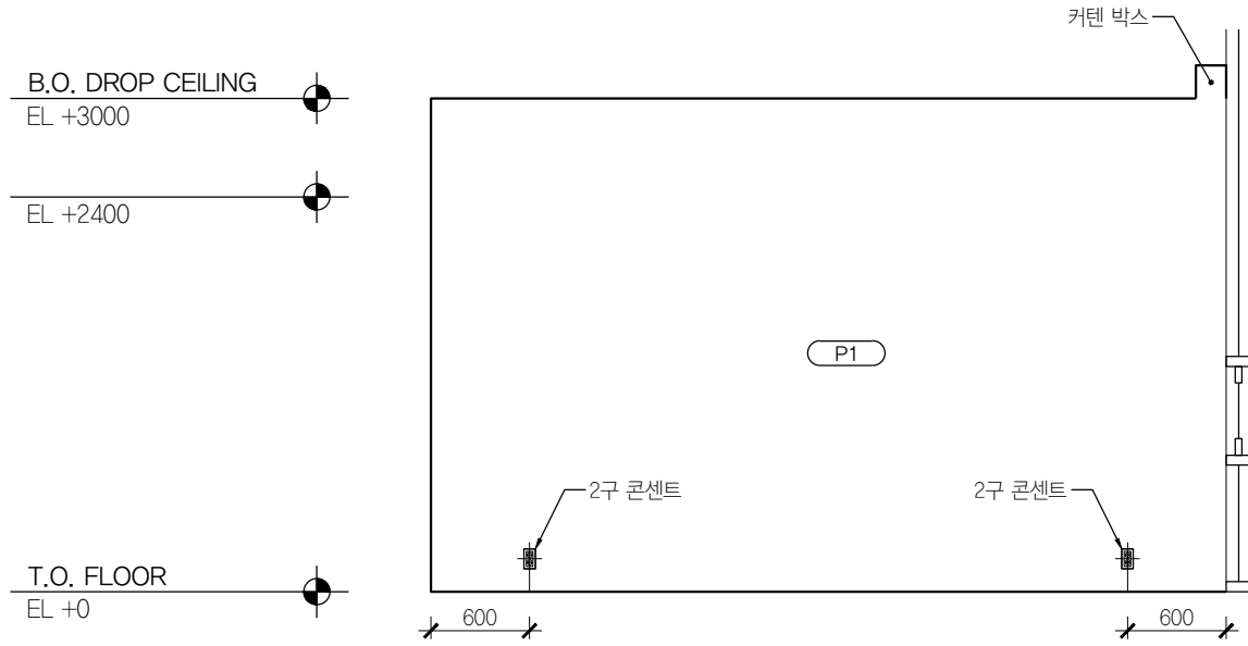
01 처장실 B109 SCALE 1:50
