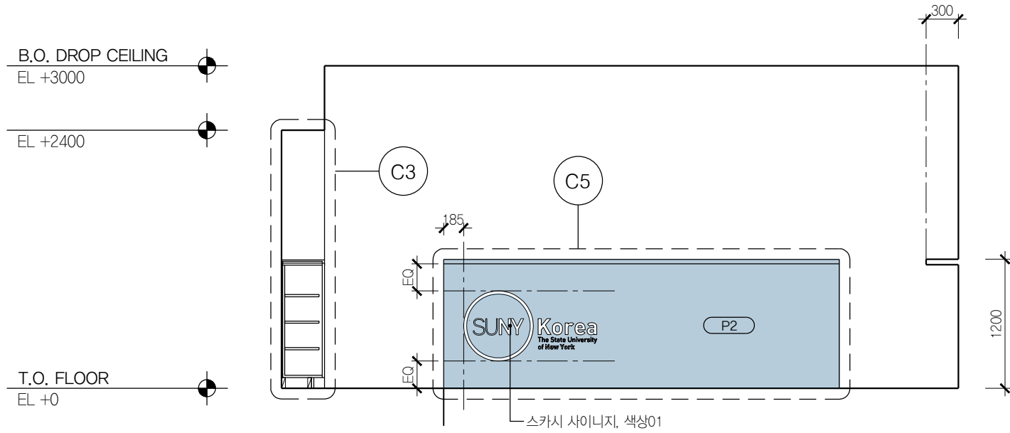
01 리셉션 B107 SCALE 1:50
