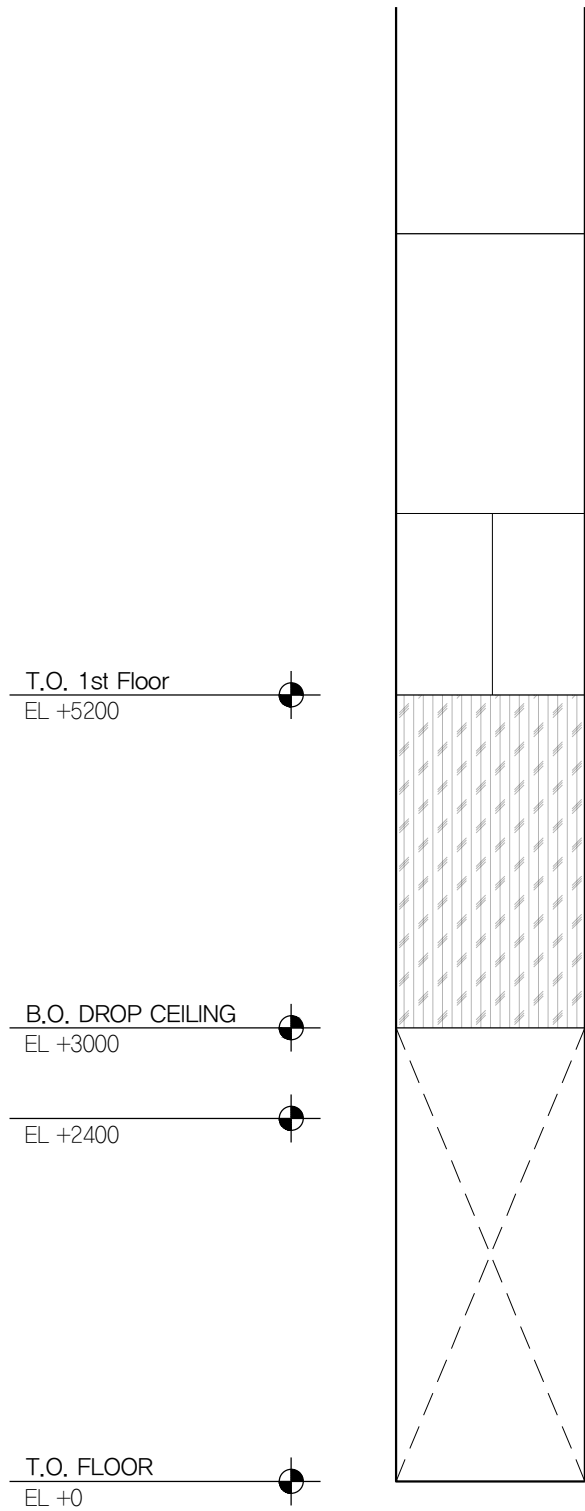
01 로비 B102 SCALE 1:50
