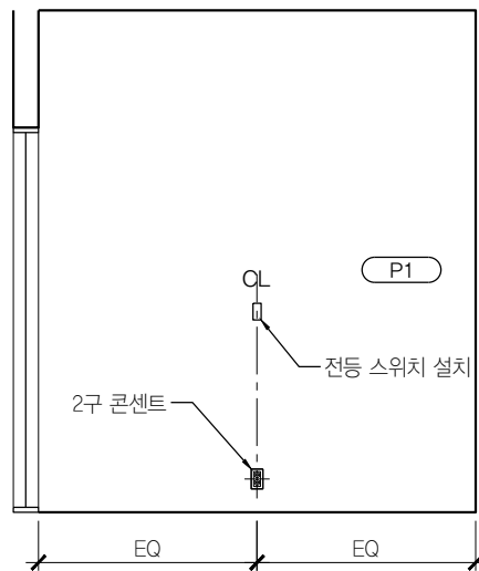
03 상담실 B110 SCALE 1:50
