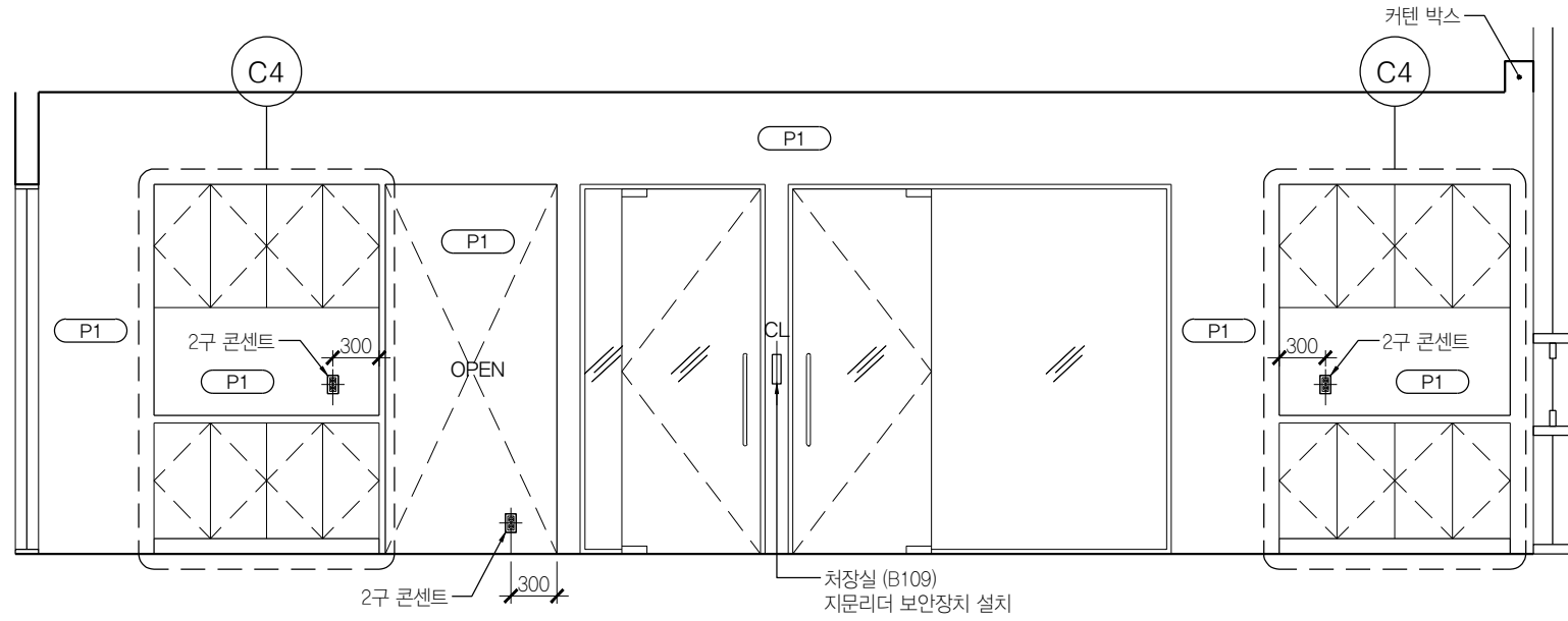
01 입학처 사무실 B112 SCALE 1:50
