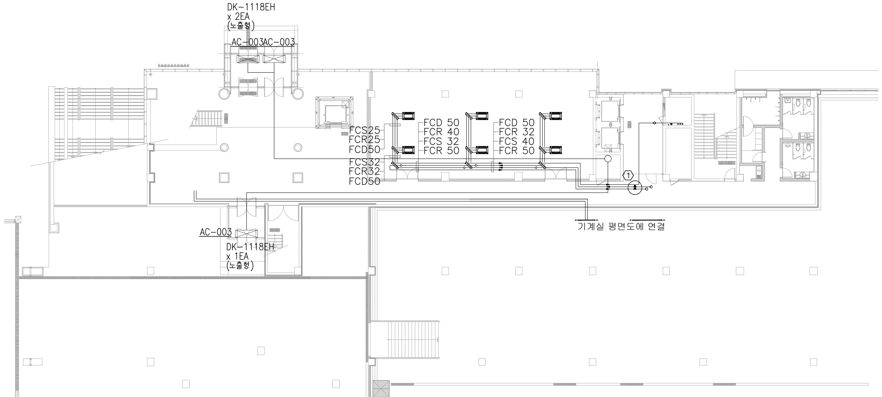
지하1층 공조배관설비 평면도(변경전) 축척 : 1 / 200
