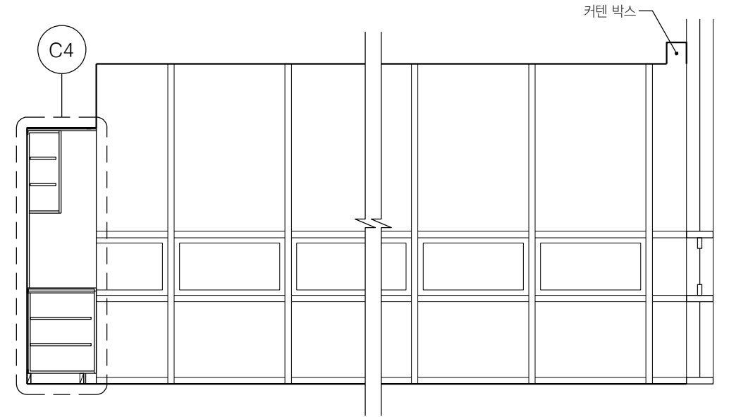
02 입학처 사무실 B112 SCALE 1:50
