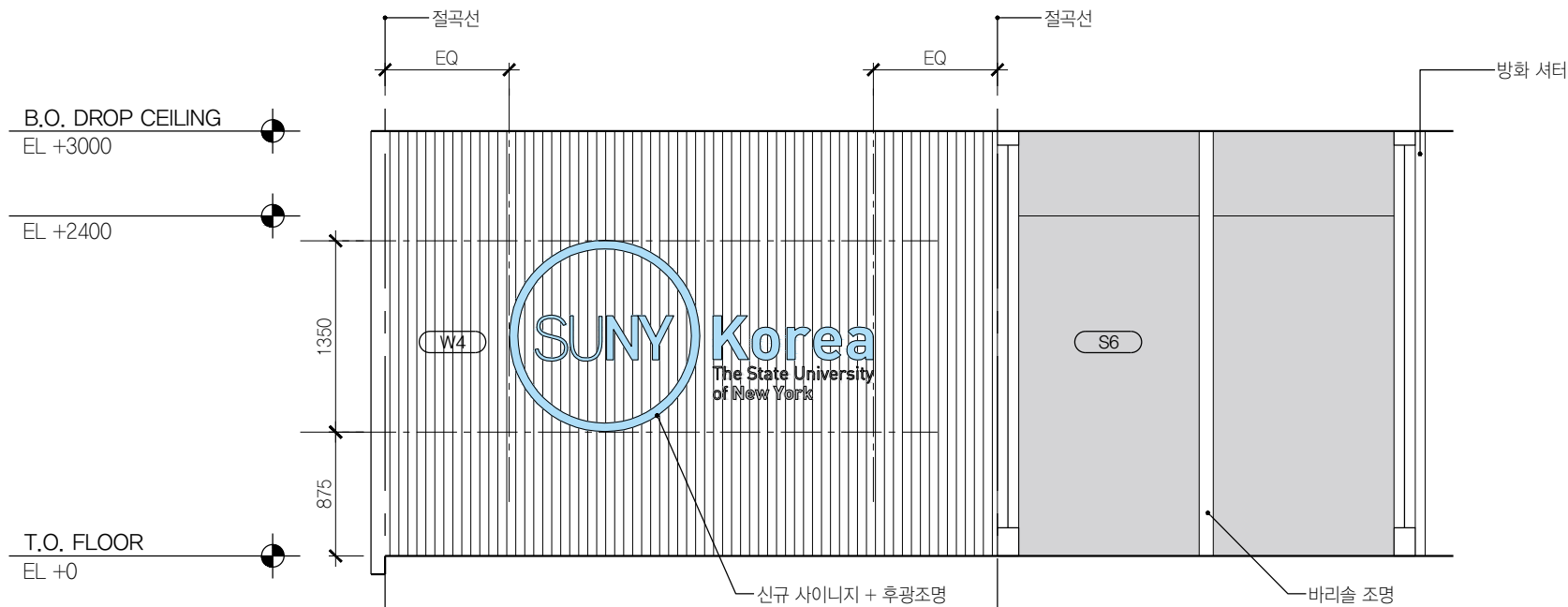
03 방풍실2 B105 SCALE 1:50
