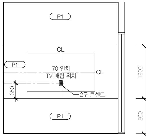
01 상담실 B110 SCALE 1:50
