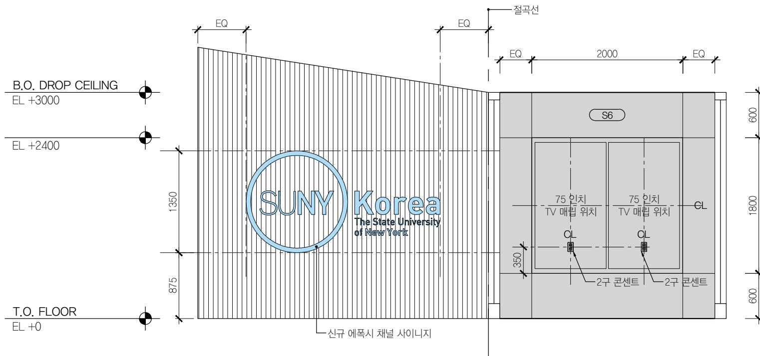
01 방풍실 B101 SCALE 1:50
