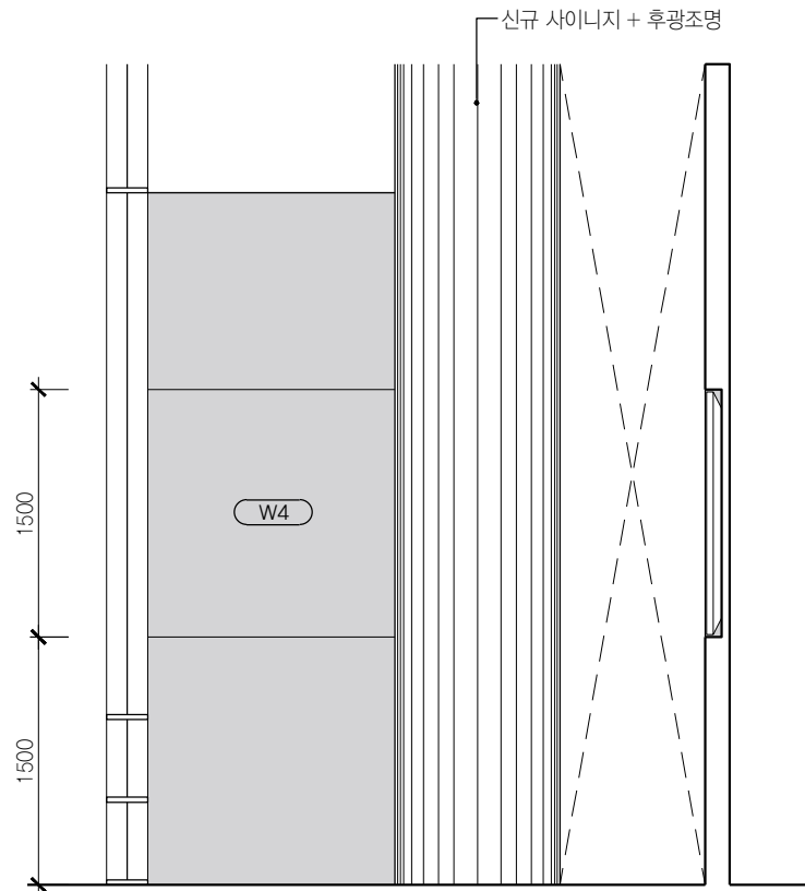
01 미팅존 B103 SCALE 1:50
