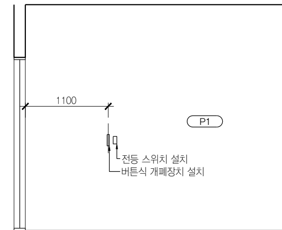
04 처장실 B109 SCALE 1:50
