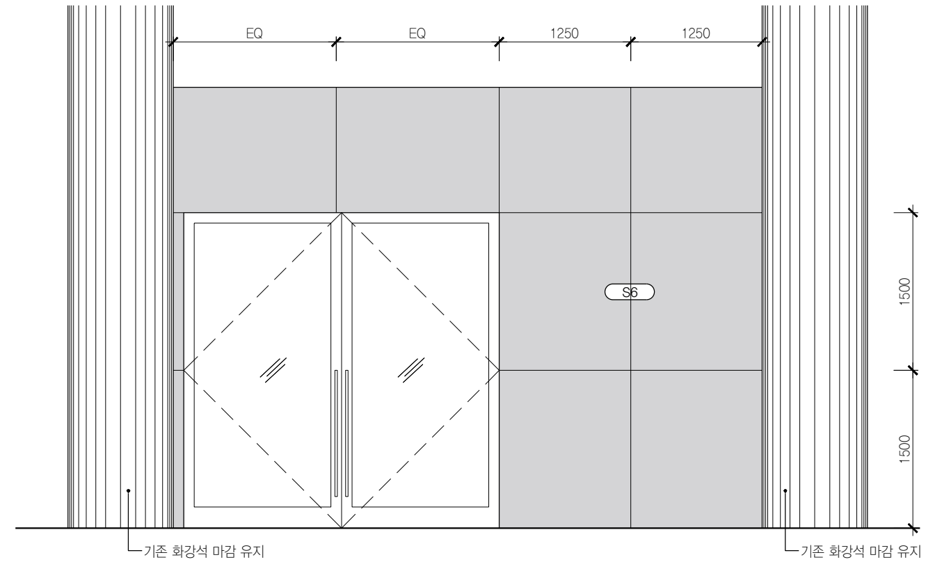
04 방풍실1 B101 SCALE 1:50
