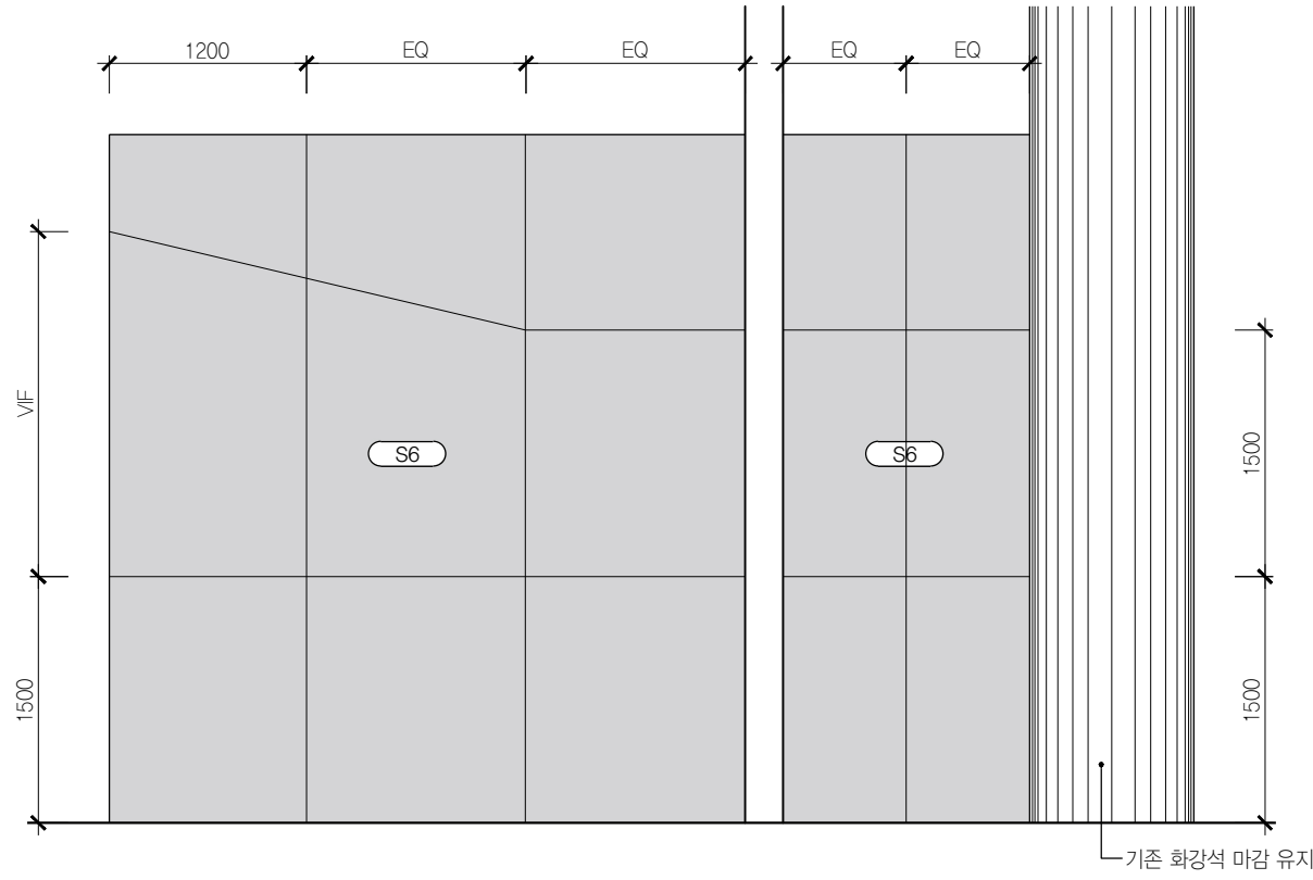
01 방풍실1 B101 SCALE 1:50
