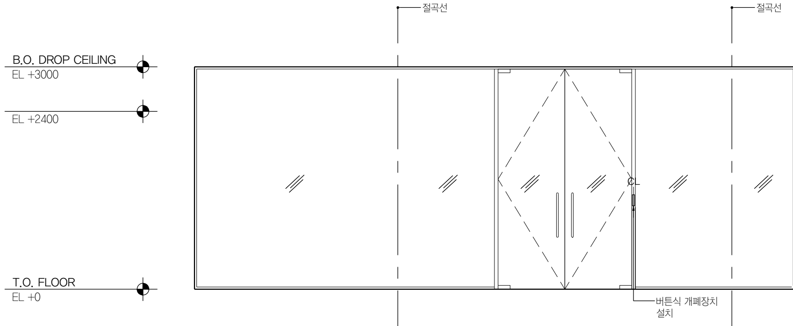
03 리셉션 B107 SCALE 1:50
