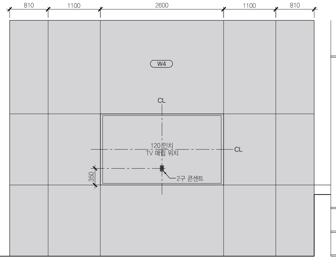
02 미팅존 B103 SCALE 1:50
