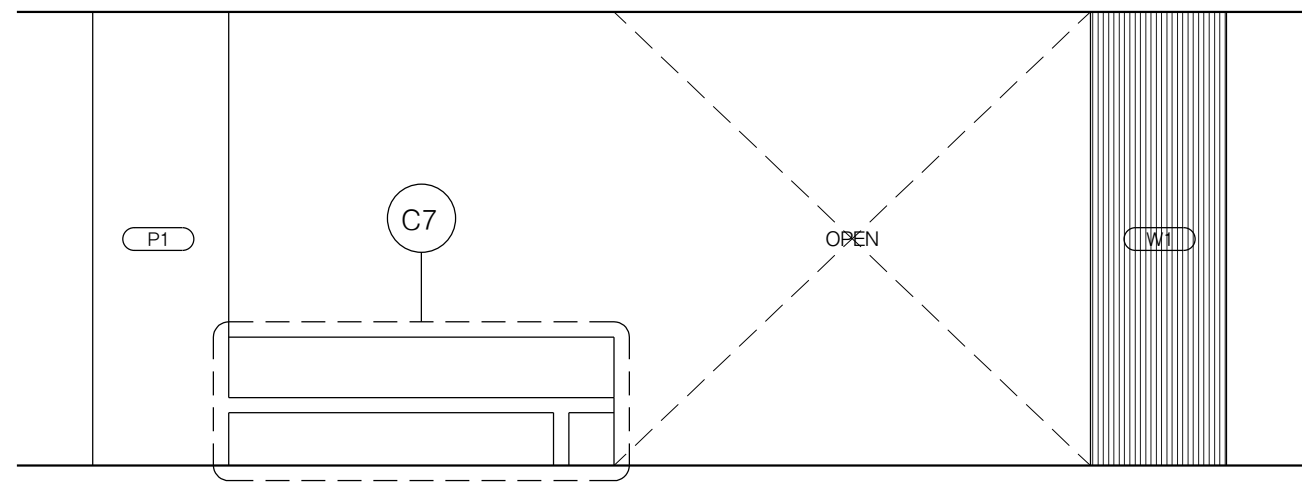
03 로비 B102 SCALE 1:50
