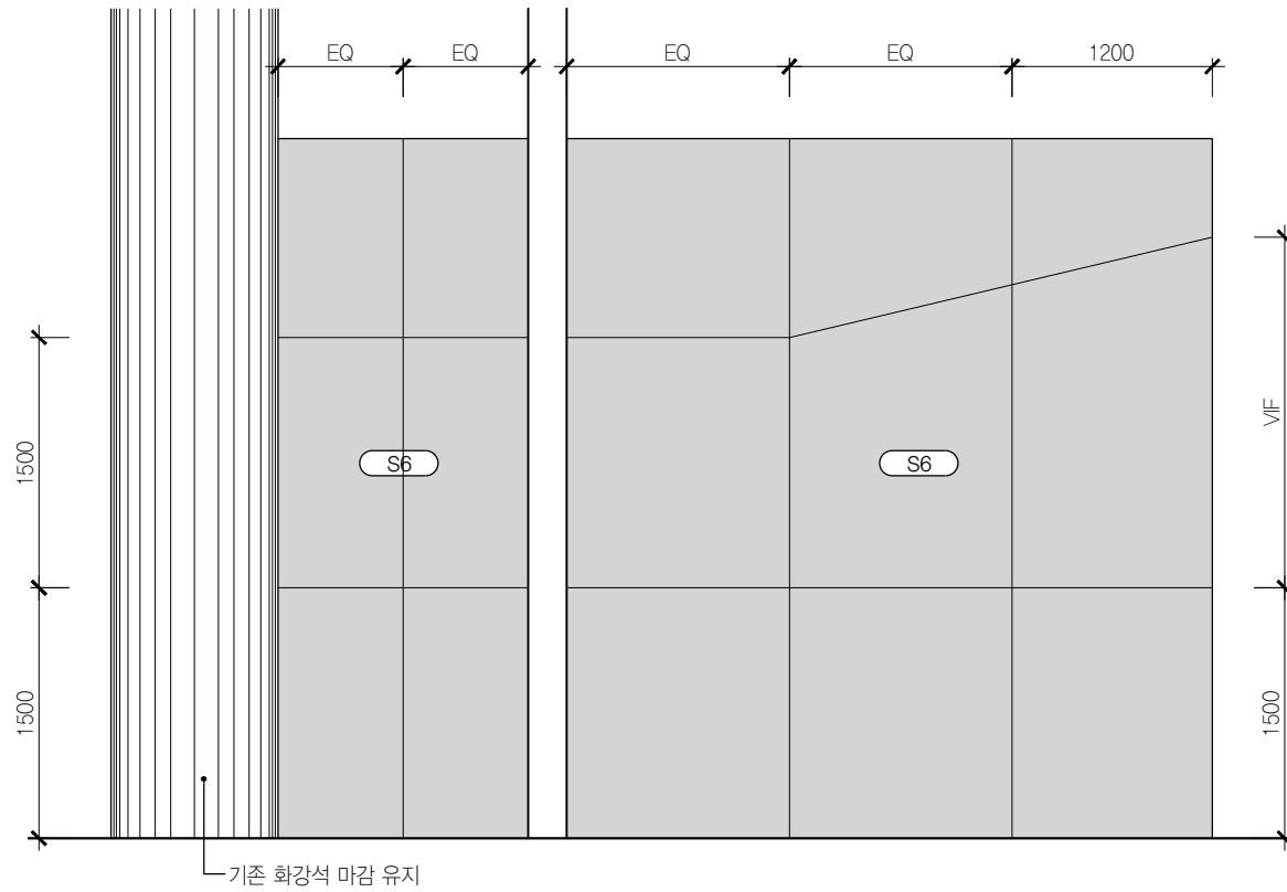
03 방풍실1 B101 SCALE 1:50
