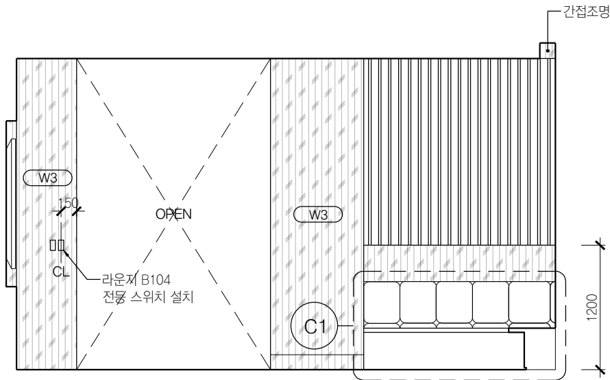
03 라운지 B104 SCALE 1:50
