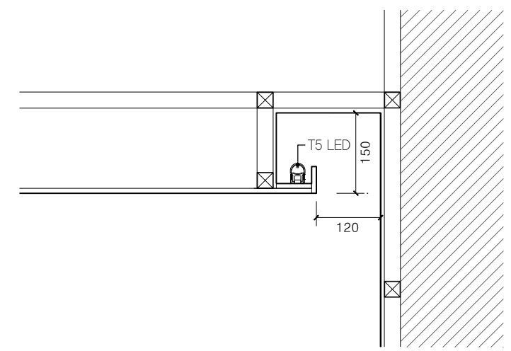
03 간접조명 상세도 SCALE 1:10
