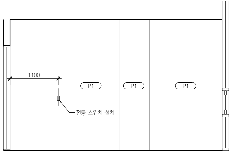
01 회의실 B108 SCALE 1:50
