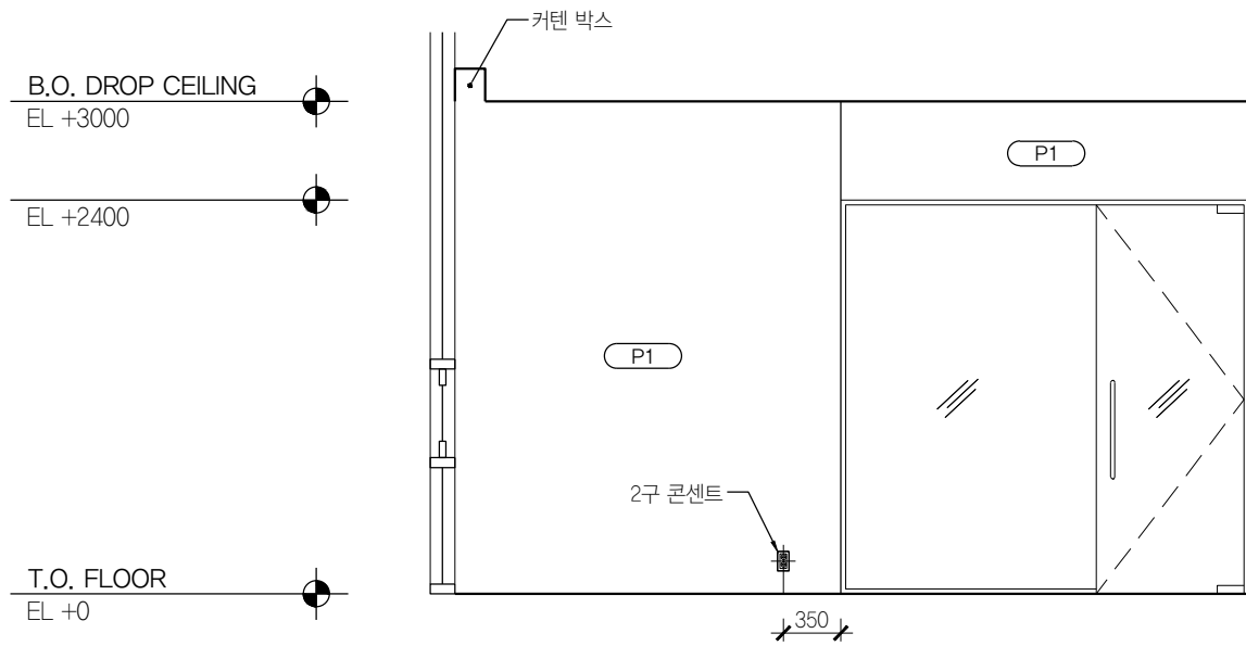
03 처장실 B109 SCALE 1:50
