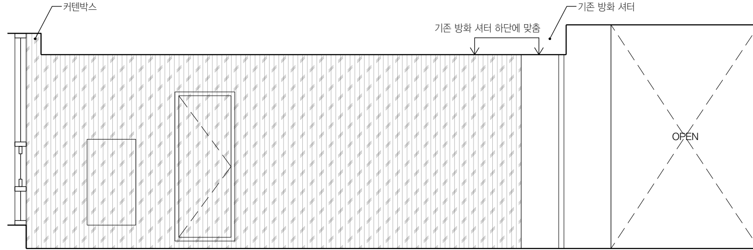
03 엘리베이터 B114 SCALE 1:50
