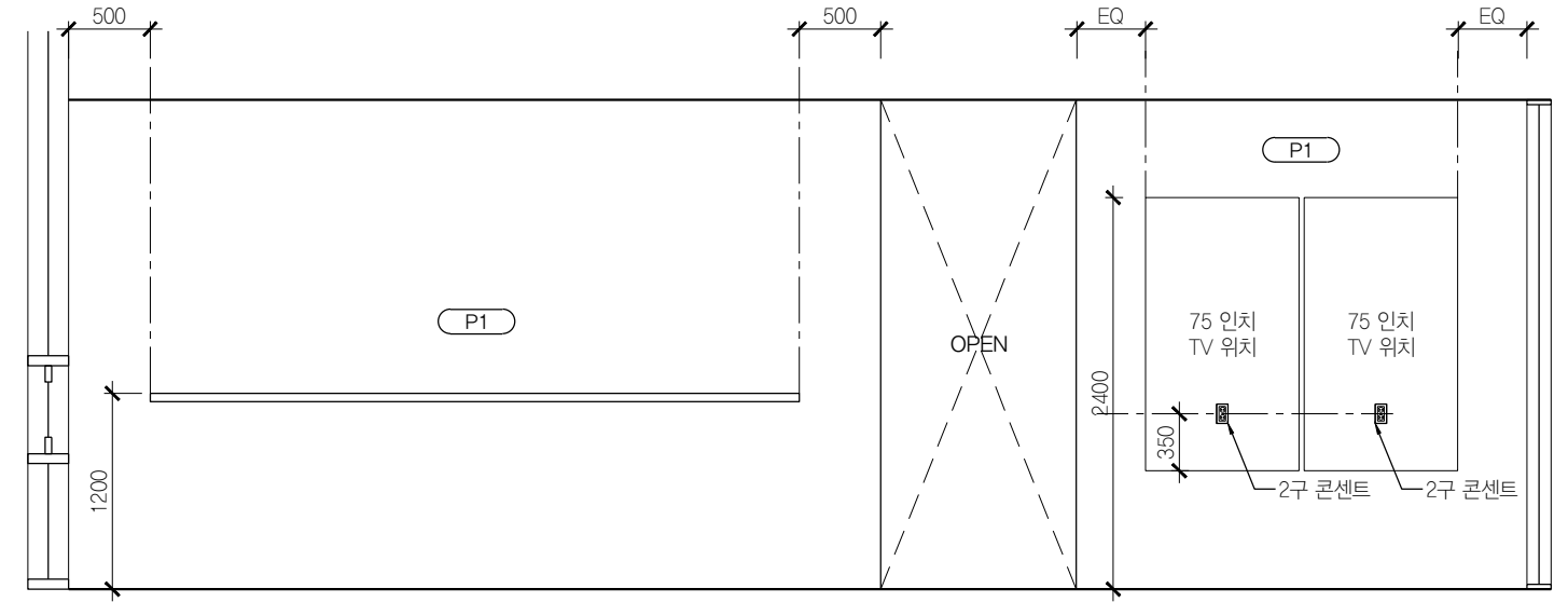
02 리셉션 B107 SCALE 1:50
