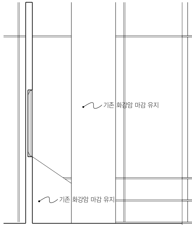
01 미팅존 B103 SCALE 1:50
